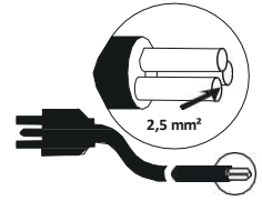
Cable alargador
